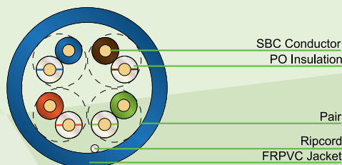
CAT5e U/UTP CMR Construction
