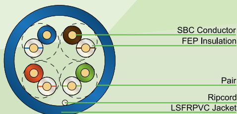
CAT5e U/UTP CMP Construction
