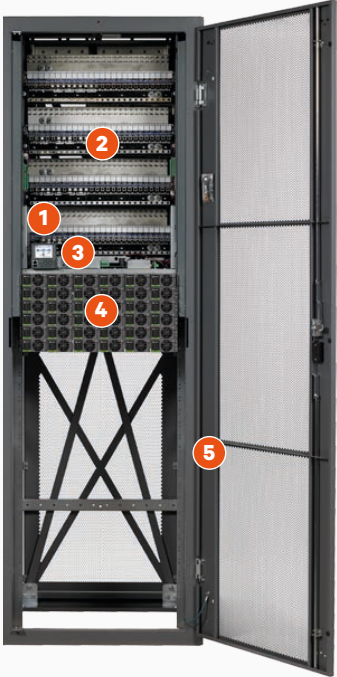
-48 VDC NetSure™ 7100
